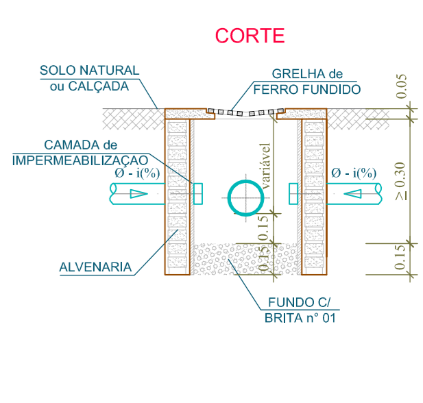
DETALHE - CAIXA de AREIA esc.: 1/25
