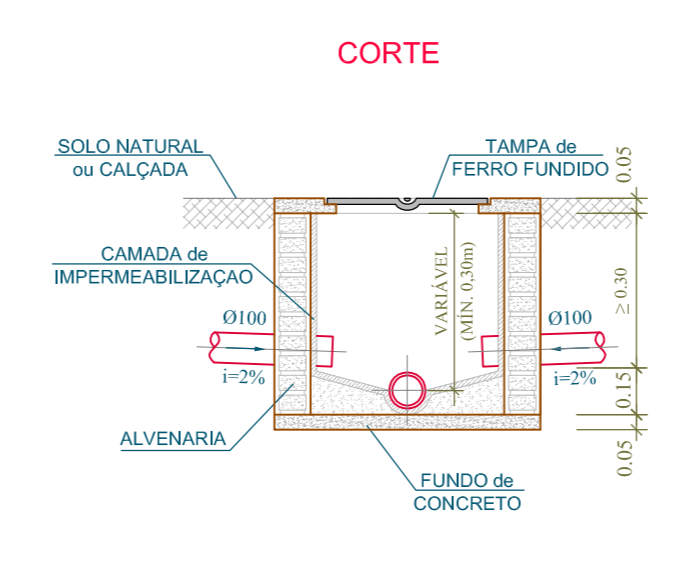
DETALHE - CAIXA de INSPEÇÃO esc.: 1/25
