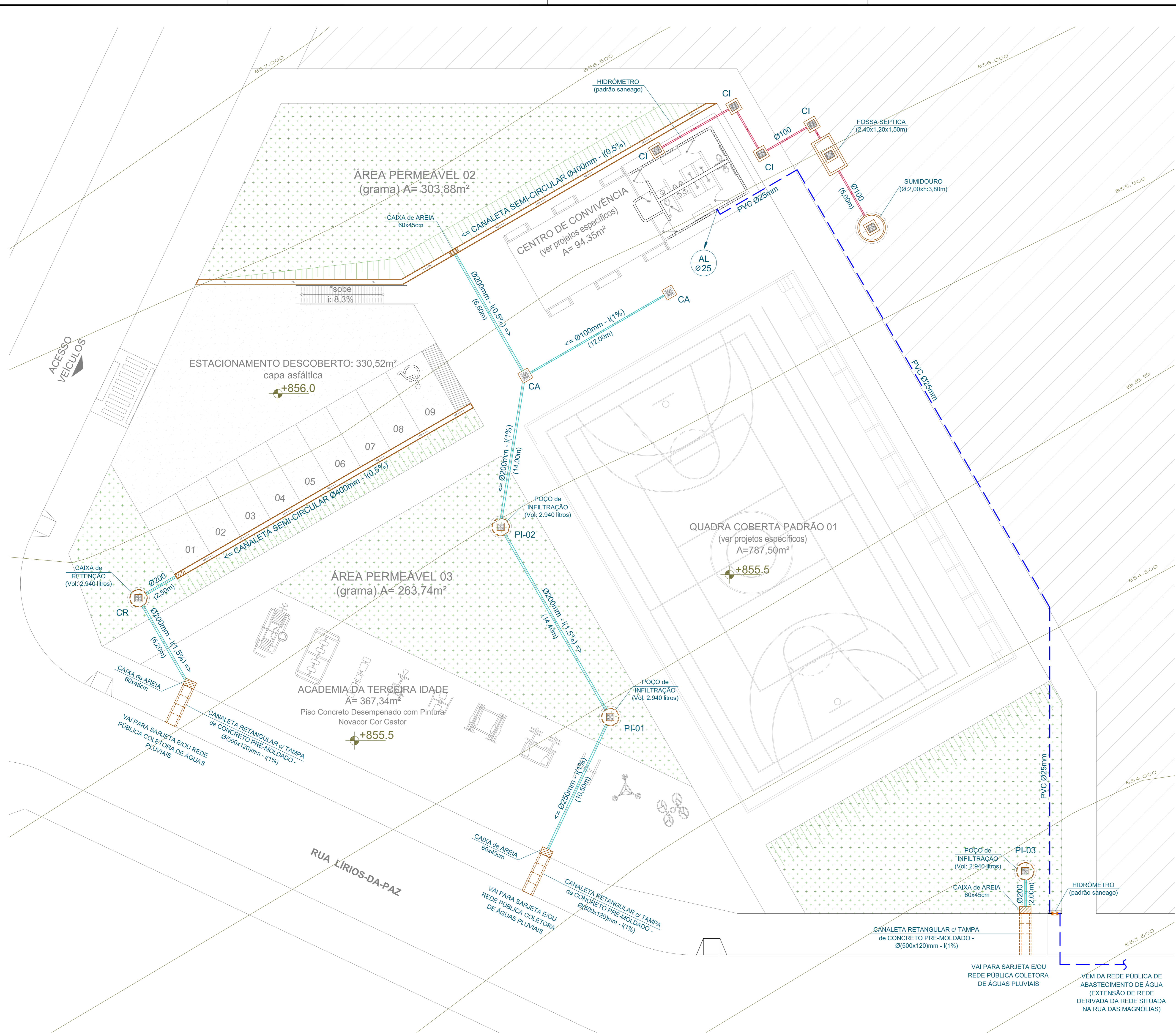
PLANTA BAIXA - IMPLANTAÇÃO (Água fria / Esgoto / Água Pluvial) esc.:1/125
