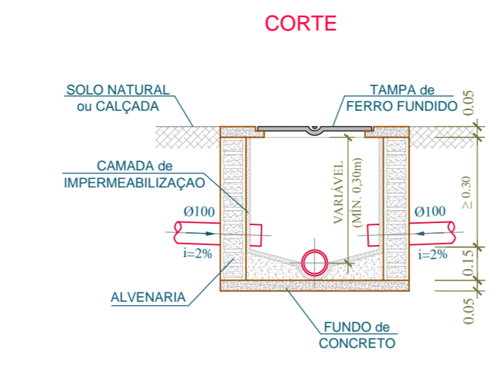
DETALHE - CAIXA de INSPEÇÃO esc.:1/25
