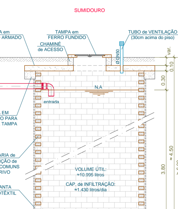
DETALHE - TANQUE SÉPTICO e SUMIDOURO(S) esc.: 1/33
