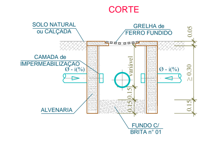
DETALHE - CAIXA de AREIA esc.:1/25
