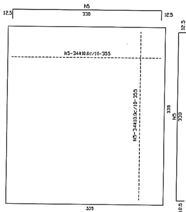
LAJE INFERIOR - ESPESSURA=15cm - FERRAGEM
