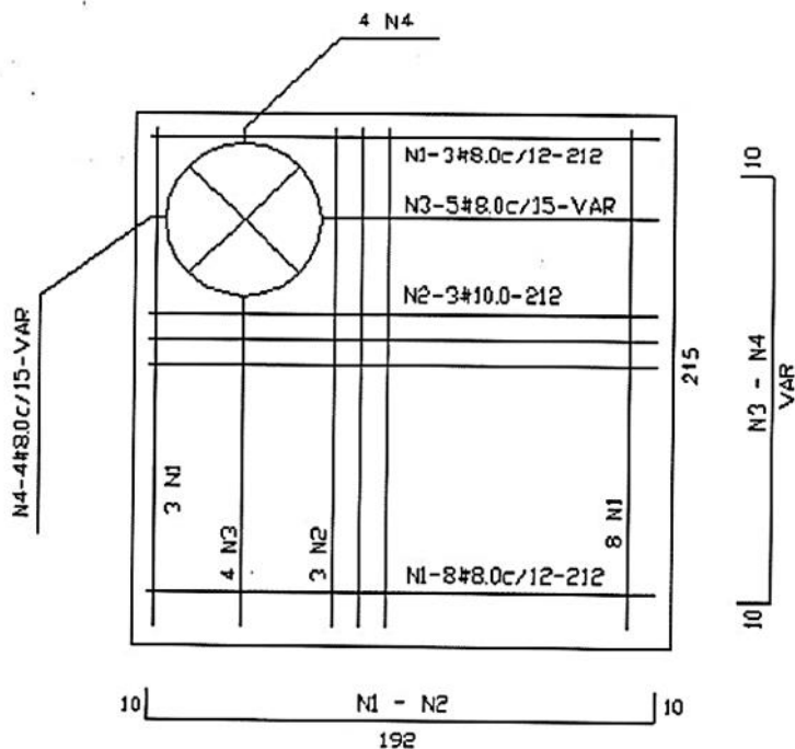
LAJE SUPERIOR - ESPESSURA=15cm - FERRAGEM
